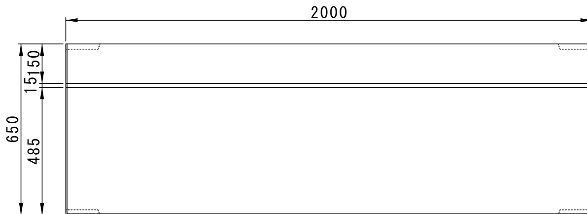
配筋図
