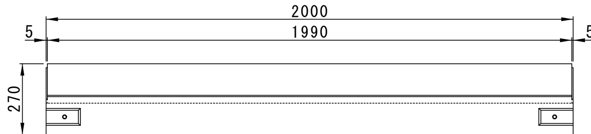
側面図
