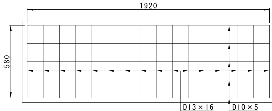
側面図
