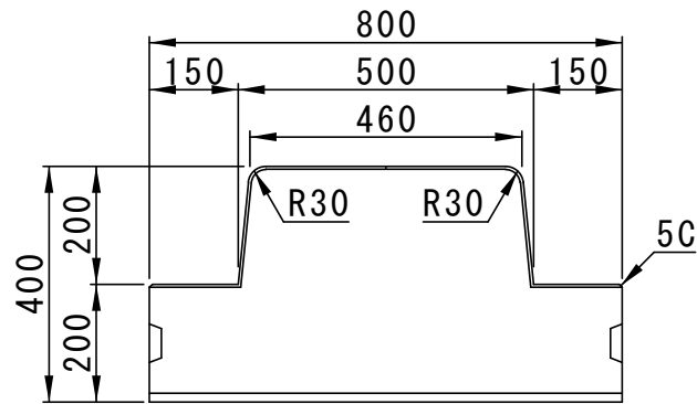
背面図
