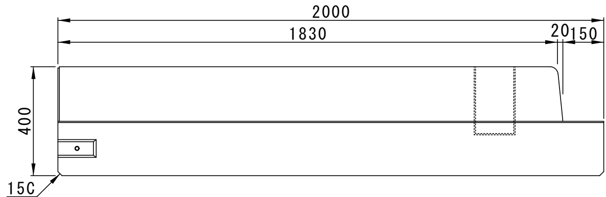
側面図
