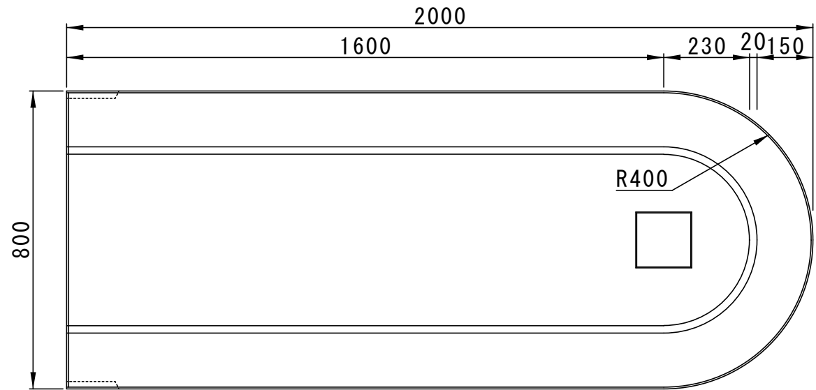
平面図
