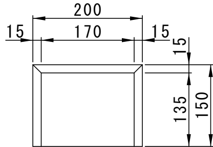
凸部詳細図
