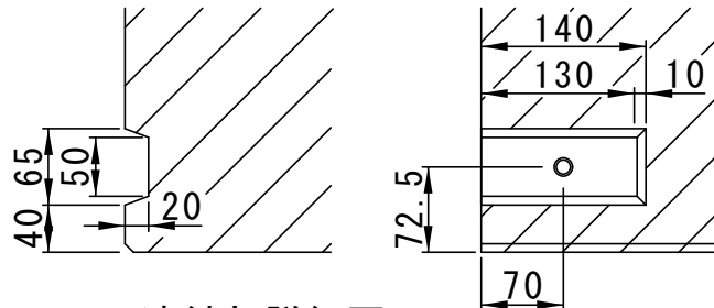
連結部詳細図
