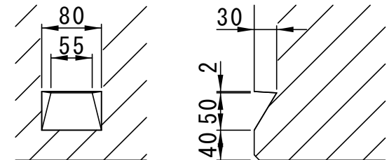
吊手部詳細図
