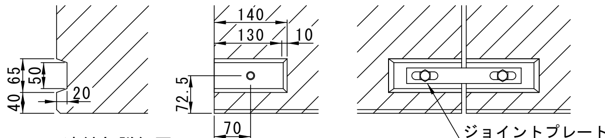
連結部詳細図
