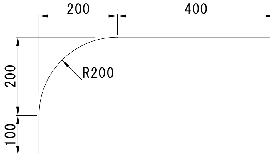
側面図
