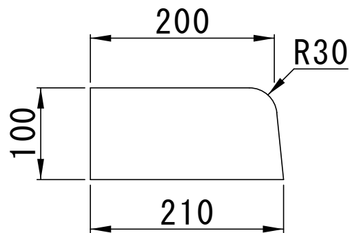
正面図
