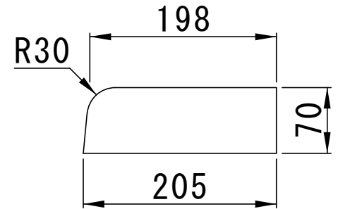
背面図
