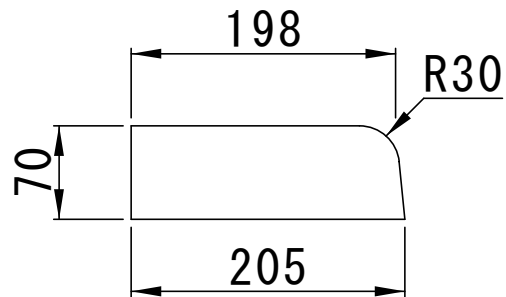
正面図
