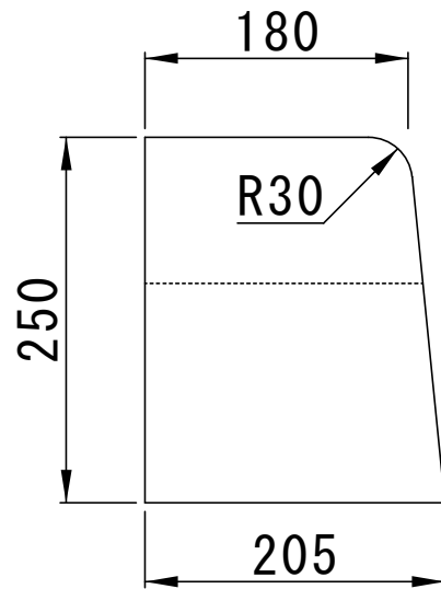
正面図
