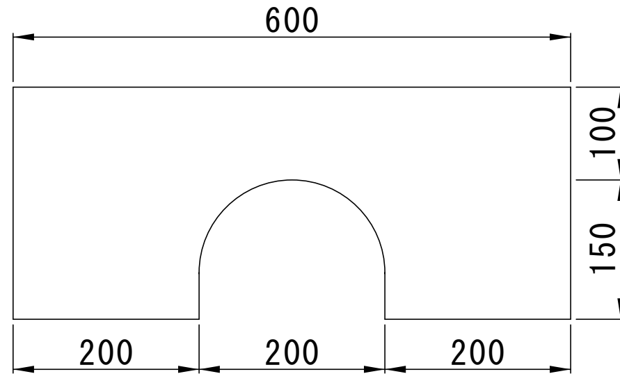
側面図
