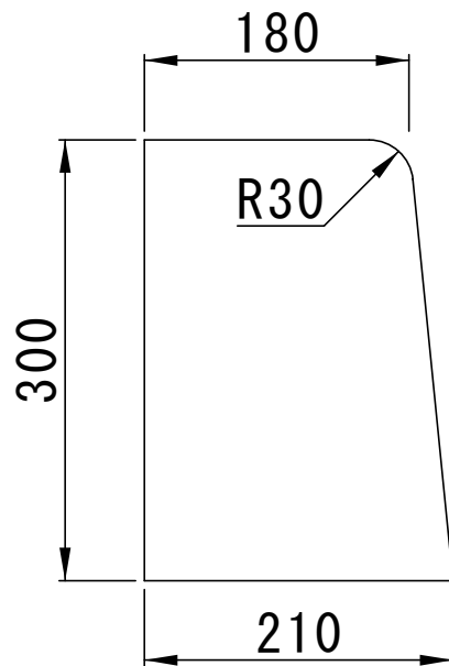
正面図
