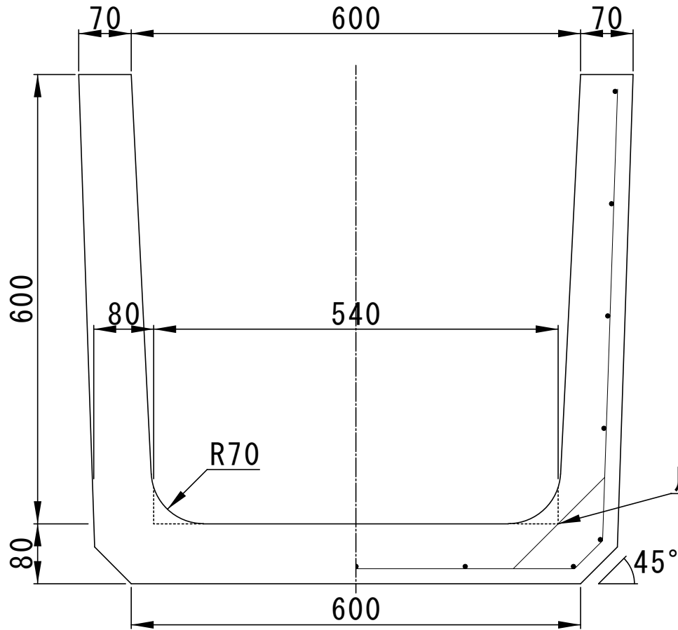
正面図
