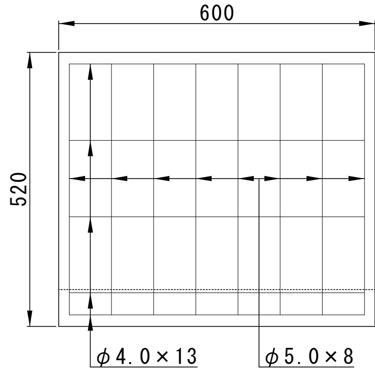
側面図
