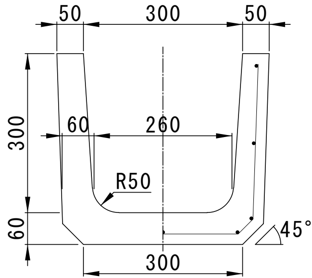
正面図
