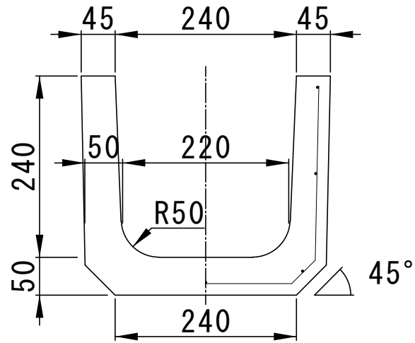
正面図
