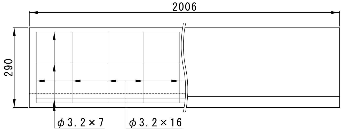
側面図
