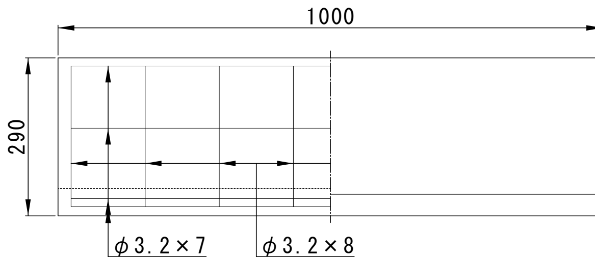
側面図
