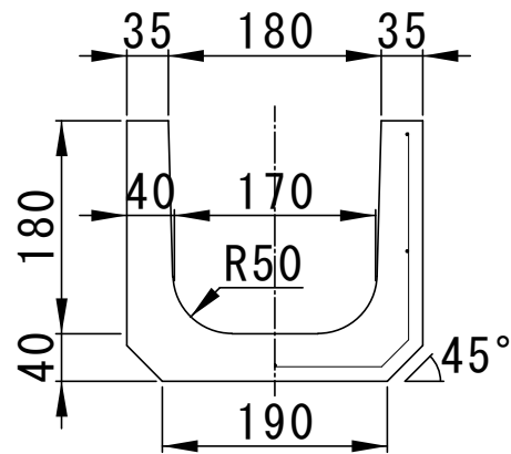
正面図
