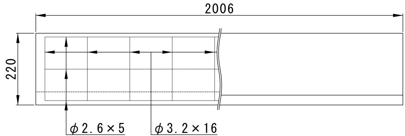
側面図
