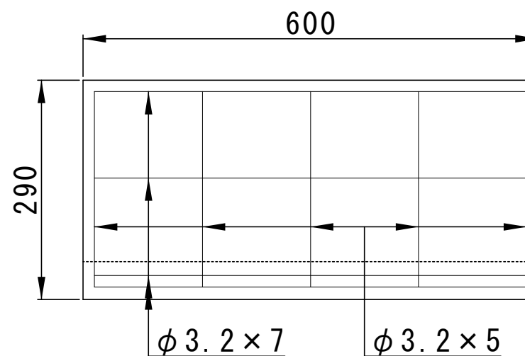
側面図
