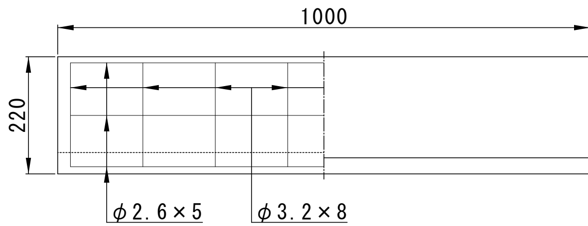
側面図
