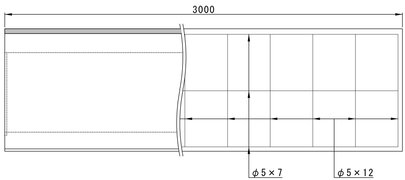
側面図
