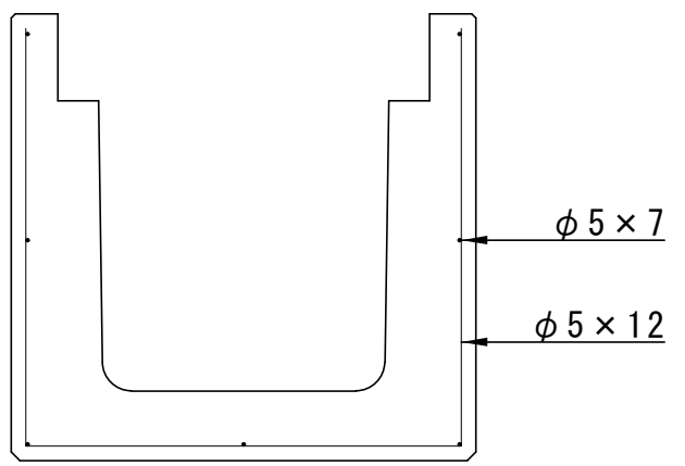
配筋図
