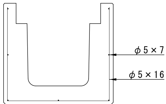
配筋図
