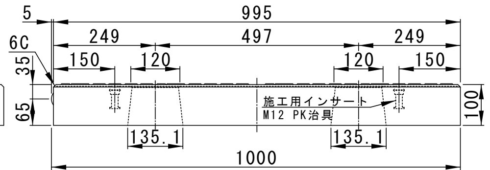
側面図
