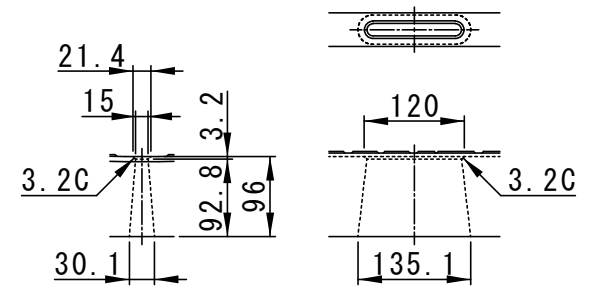
水抜孔詳細図
