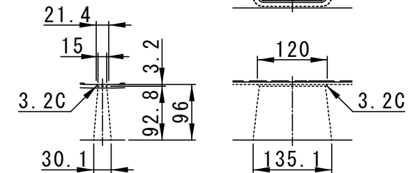
水抜孔詳細図
