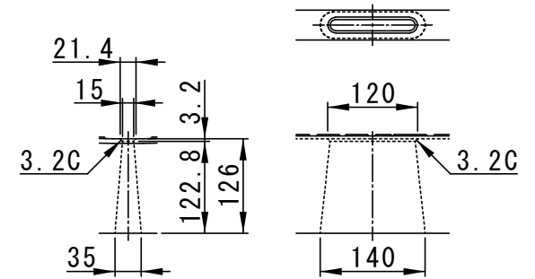
水抜孔詳細図
