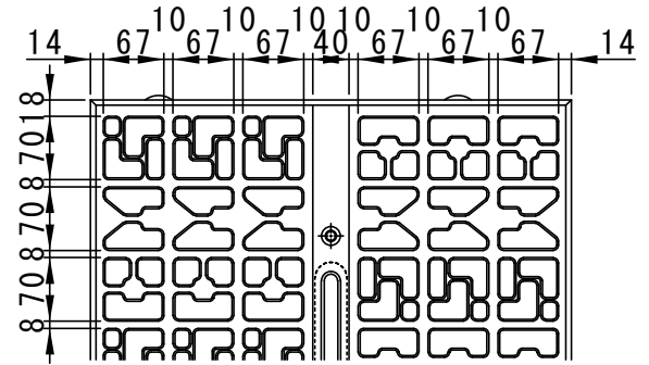
CMS 模様部詳細図
