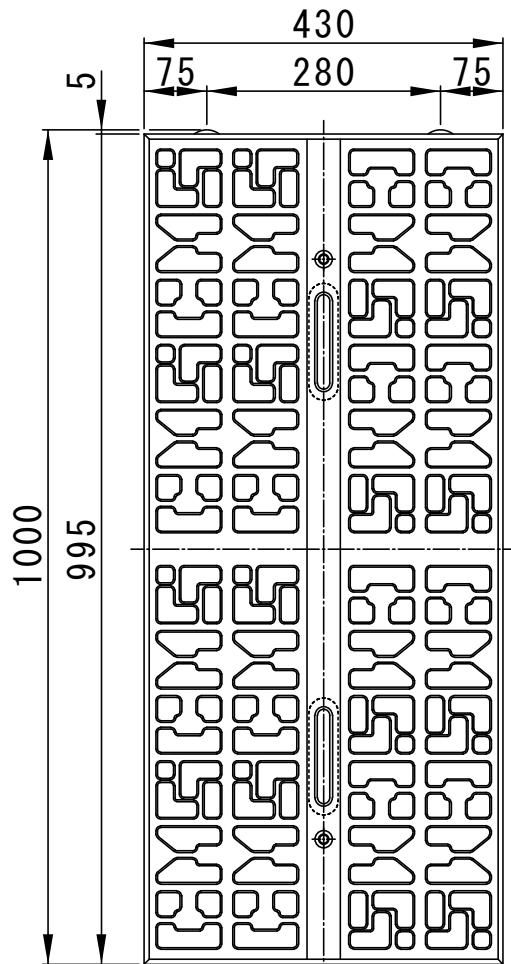
平面図
