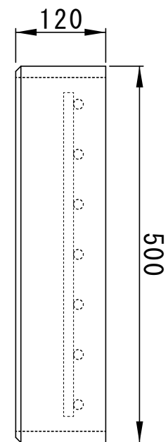
側面図
