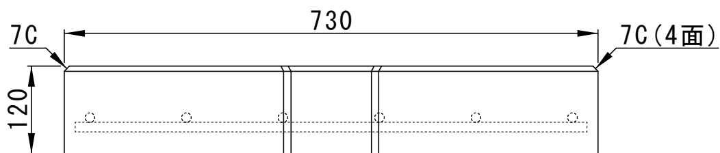
正面図
