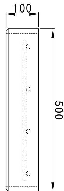
側面図
