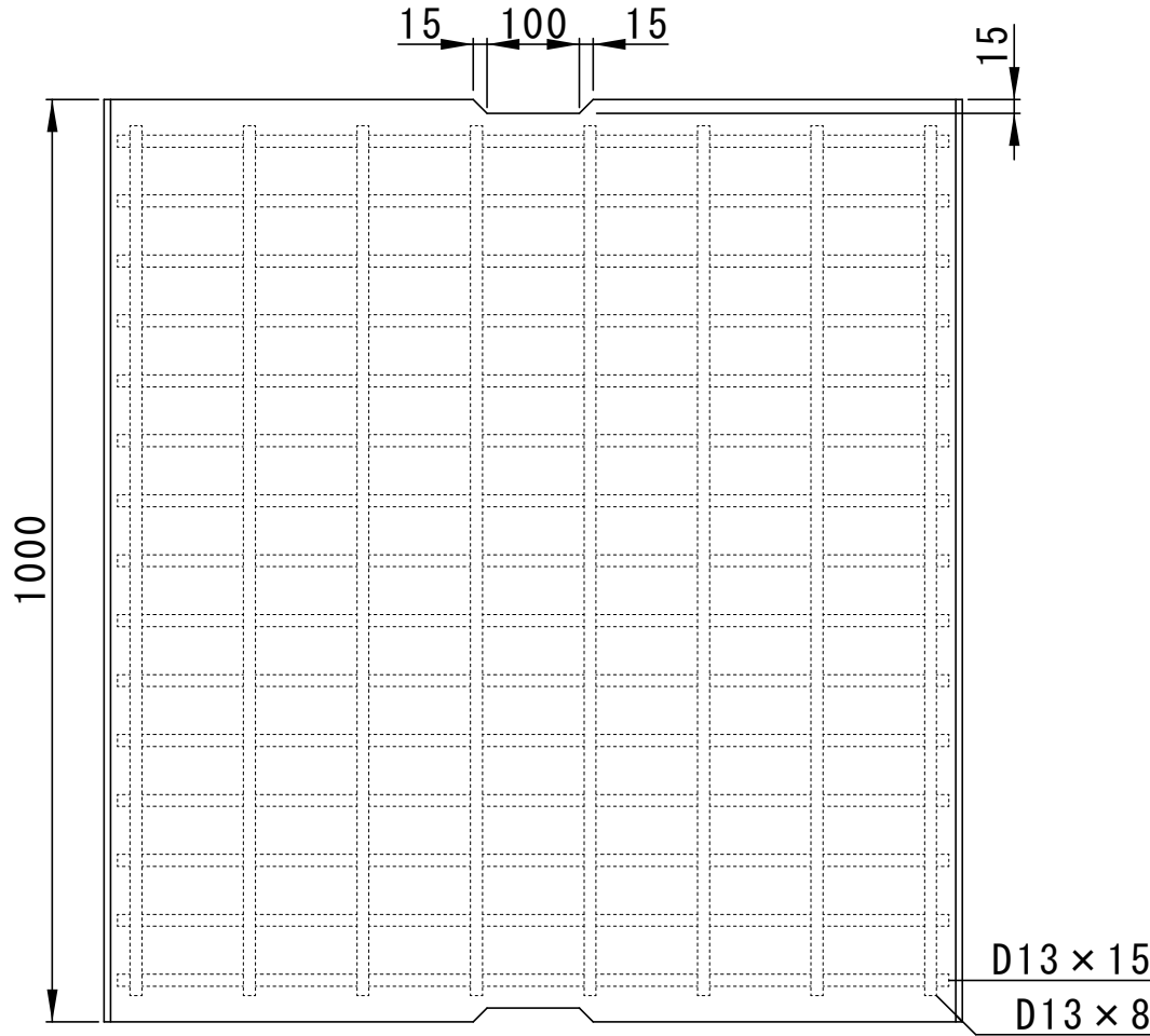
平面図
