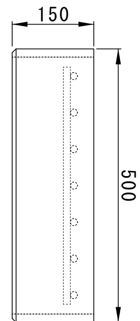
側面図
