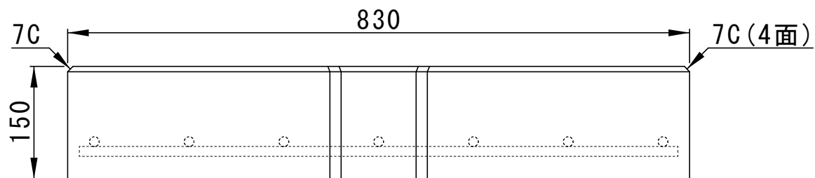
正面図
