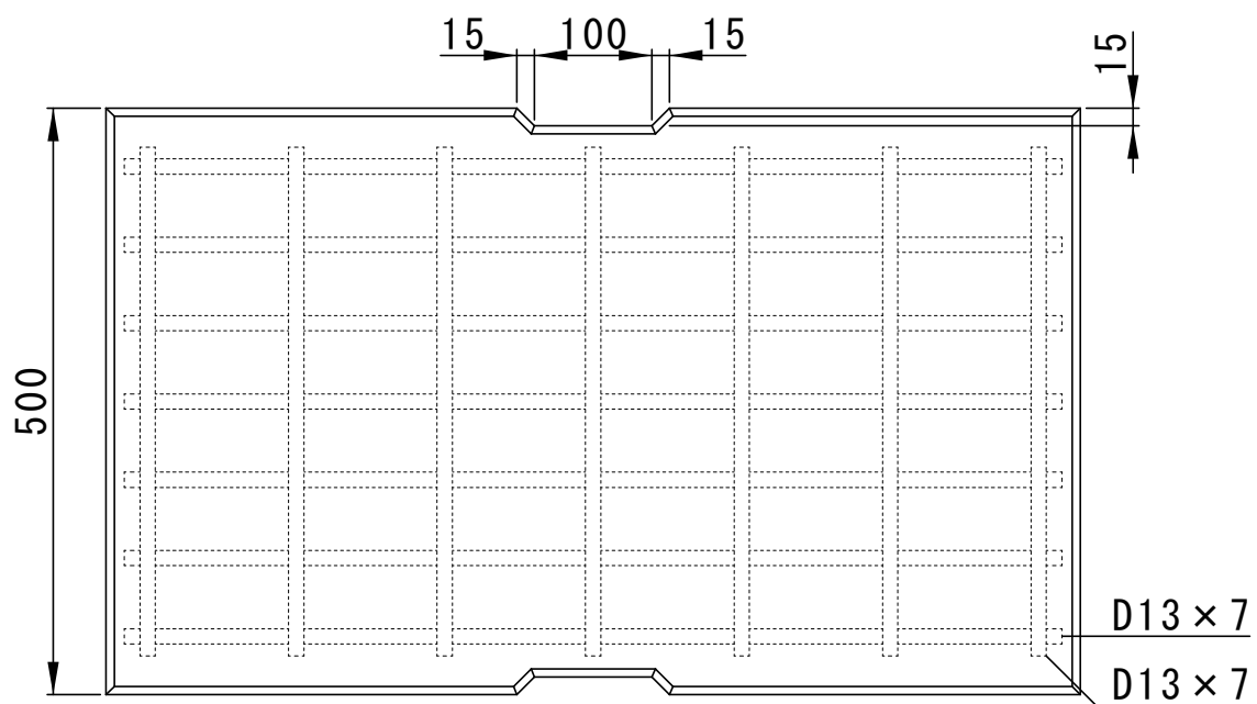
平面図
