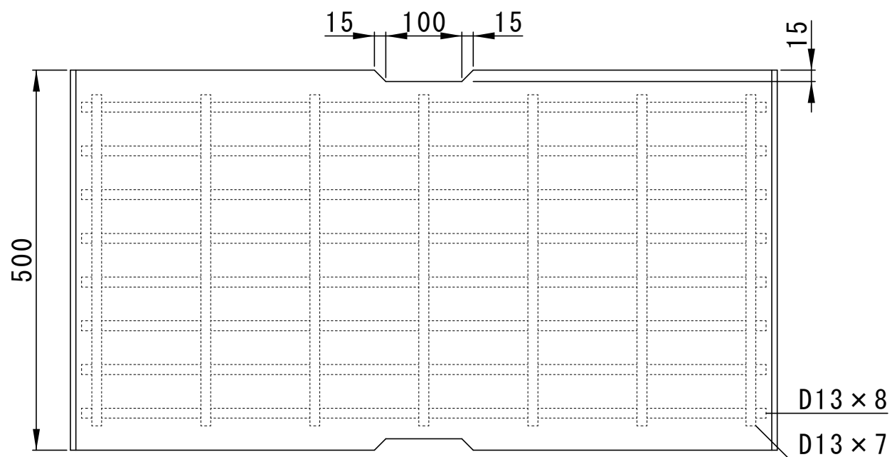
平面図
