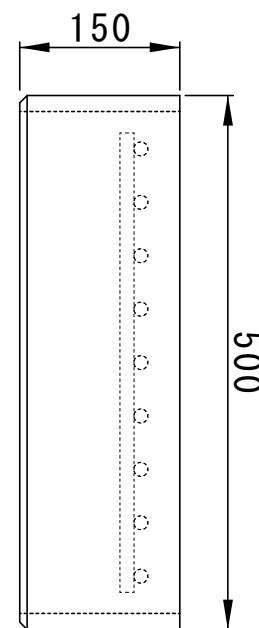
側面図
