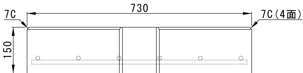
正面図
