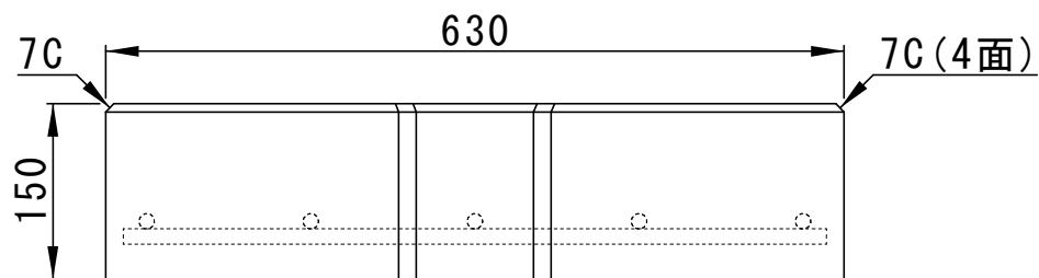
正面図
