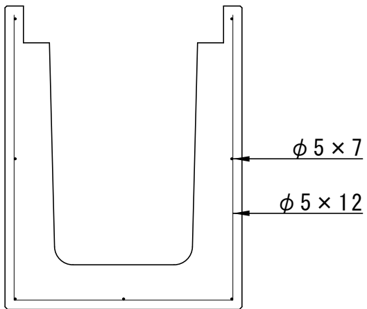
配筋図
