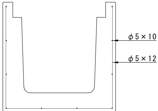
配筋図
