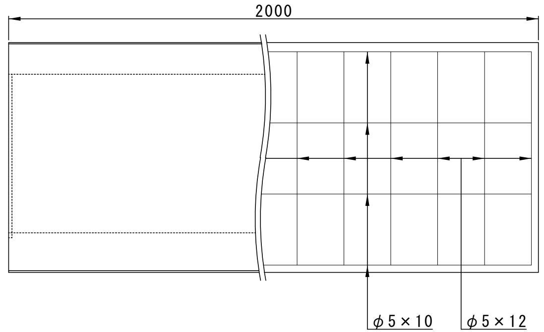
側面図
