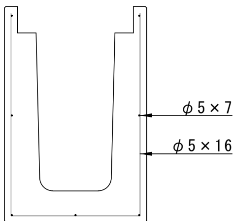
配筋図
