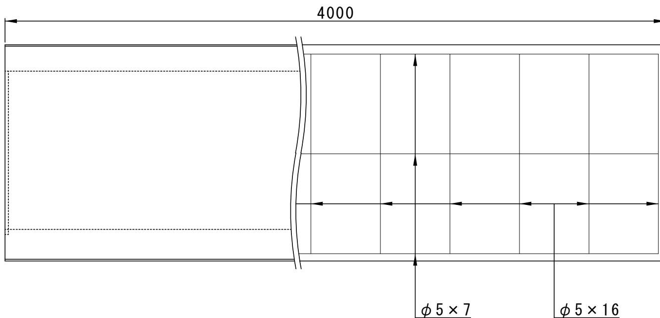
側面図
