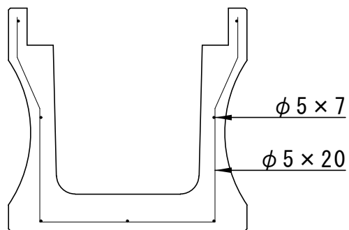
配筋図
