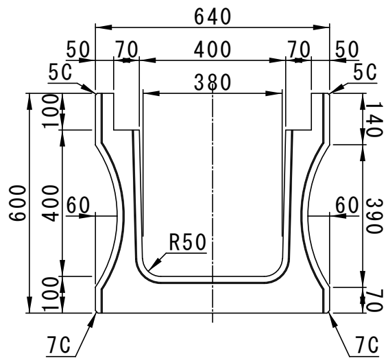
正面図
