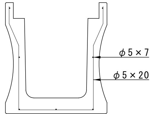
配筋図
