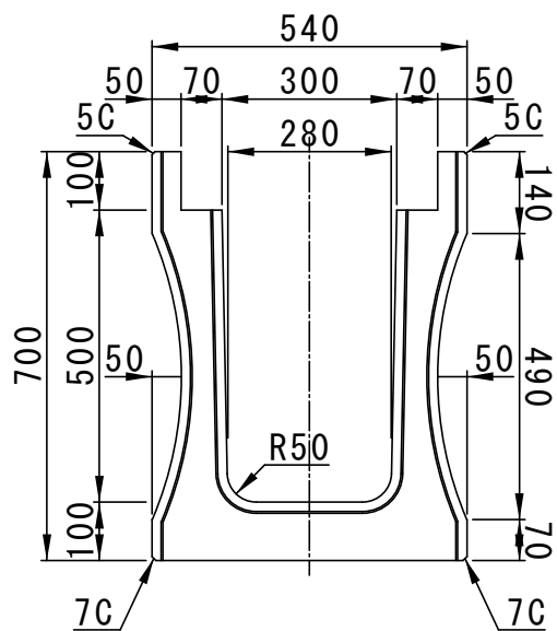
正面図
