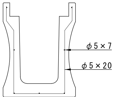
配筋図
