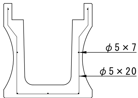
配筋図
