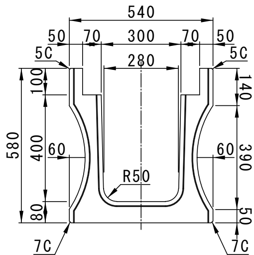
正面図
