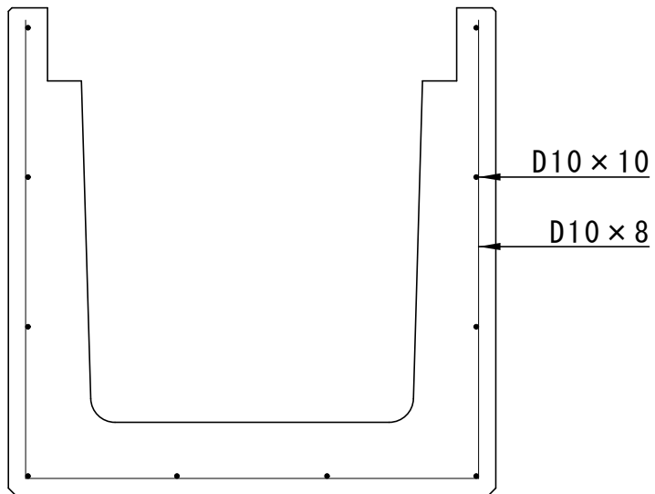
配筋図
