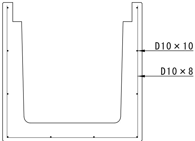
配筋図
