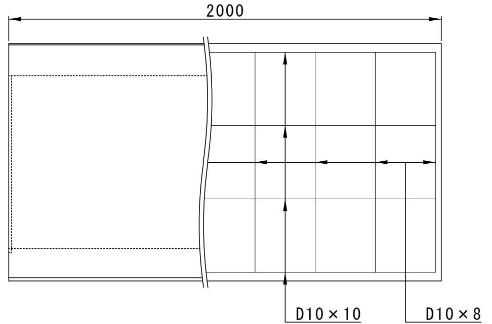
側面図
