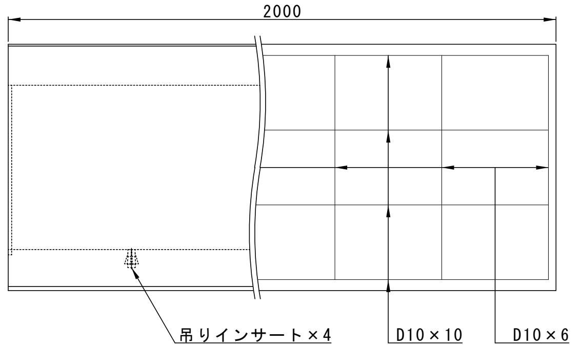
側面図
