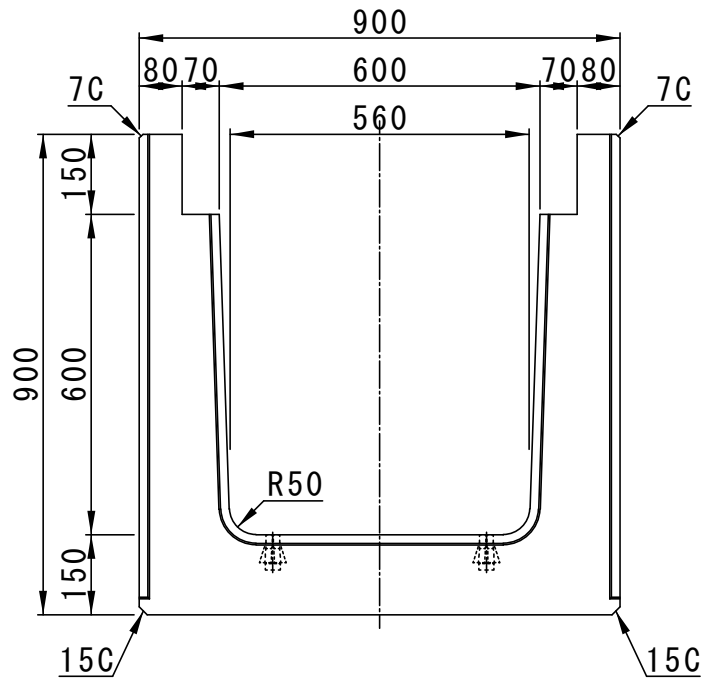
配筋図
