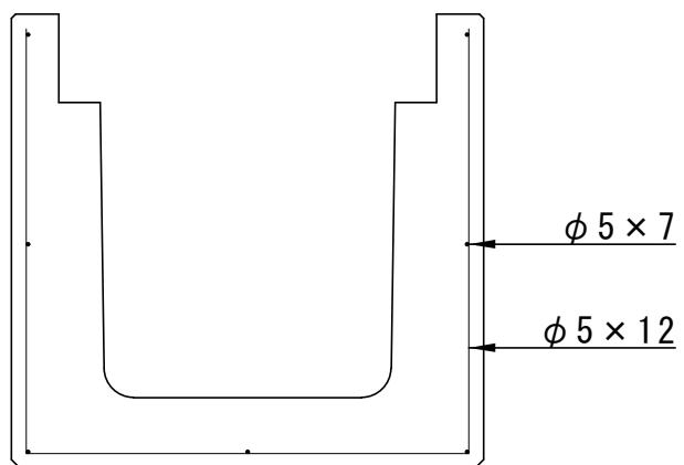
配筋図
