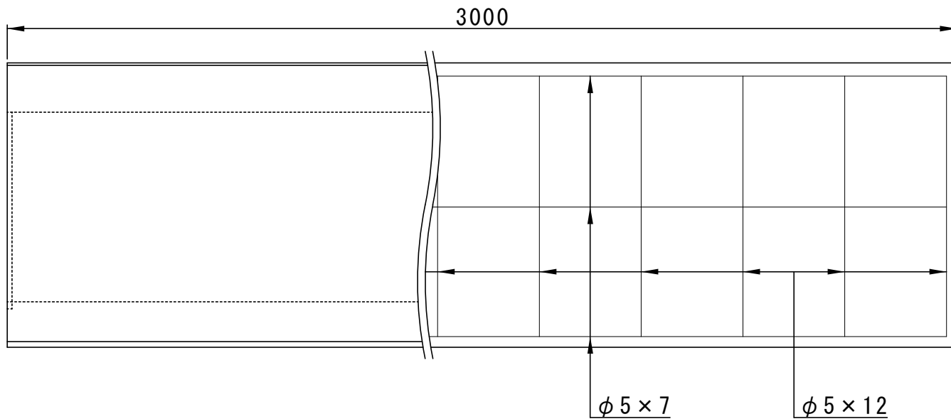
側面図
