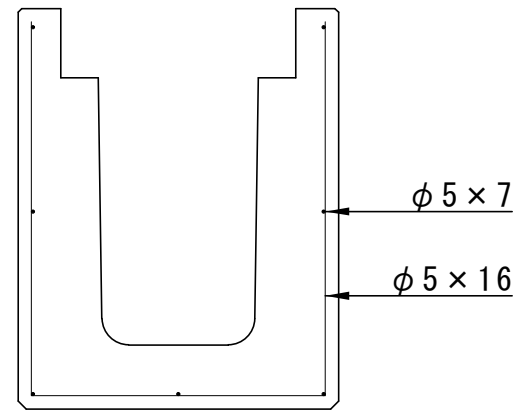
配筋図
