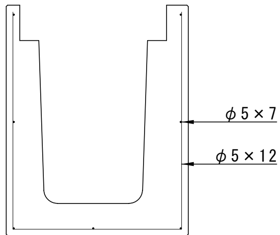
配筋図
