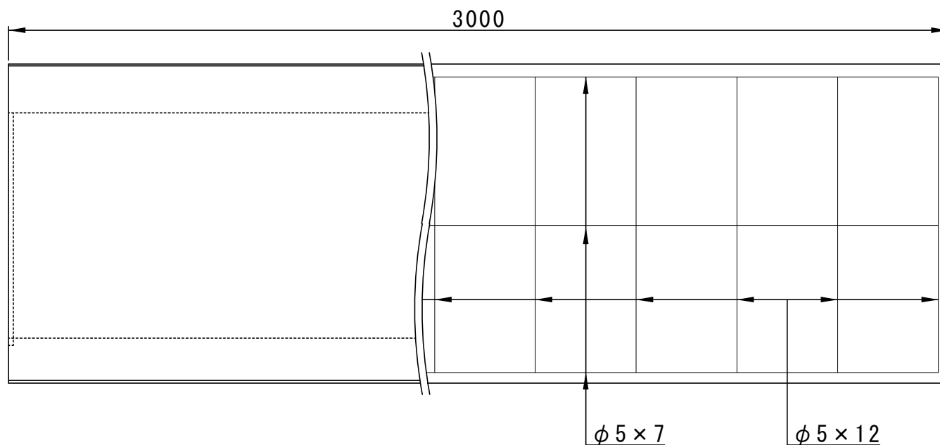
側面図
