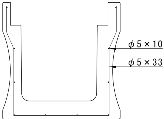
配筋図
