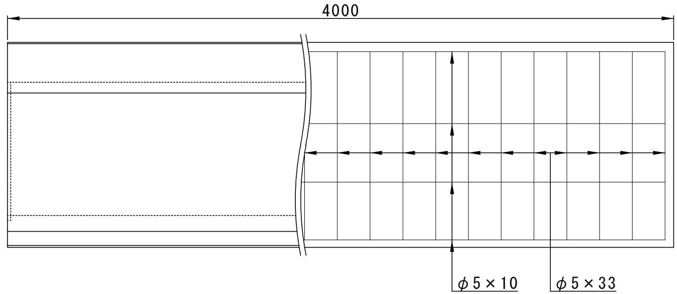
側面図
