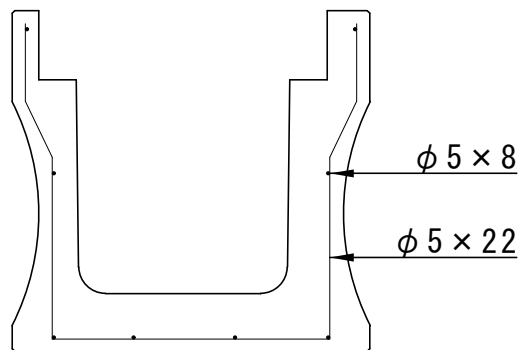
配筋図
