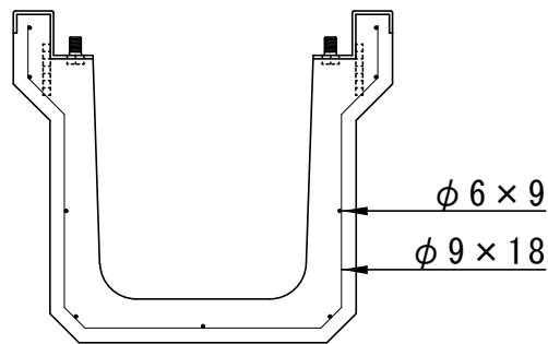
配筋図
