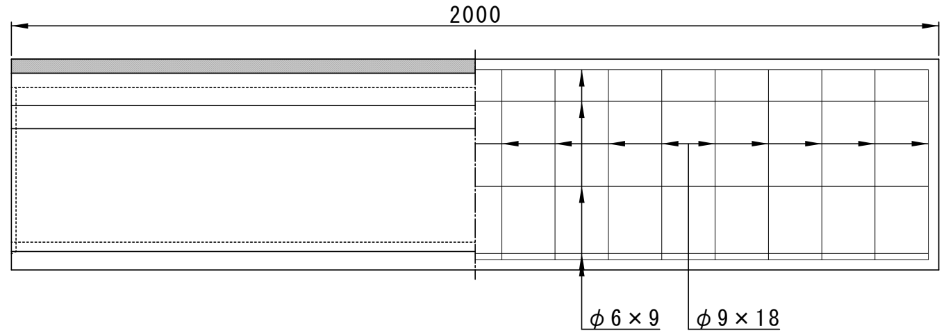
側面図
