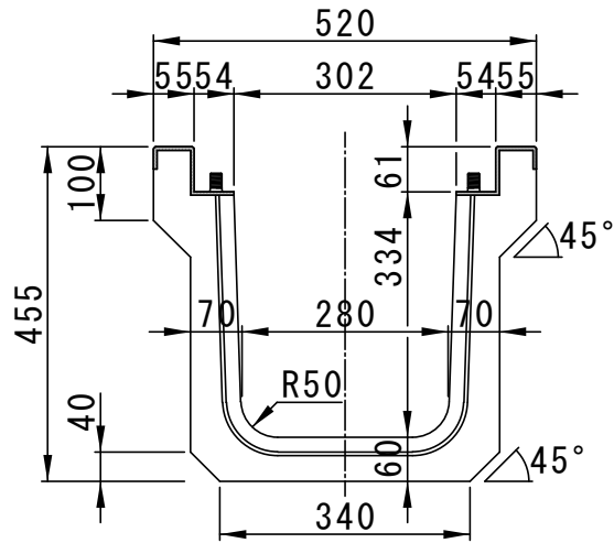
正面図
