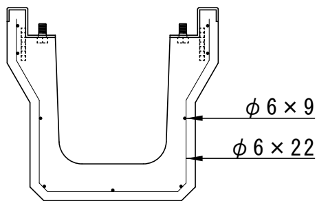
配筋図
